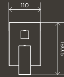
Inbouw mengkraan met omstel klein
